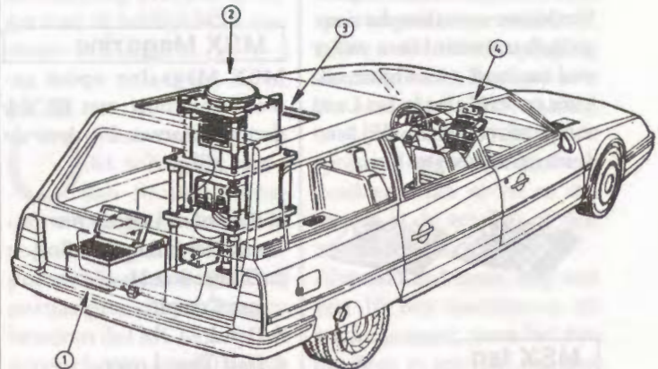
Het opnamesysteem van Frank, gemonteerd in een bestelauto. Betekenis van de cijfers: 1. computer voor registratie van de stand van het platform; 2. 'fish eye'-optiek; 3. stabilisatieplatform; 4. computer voor meldingen van en aan chauffeur.
