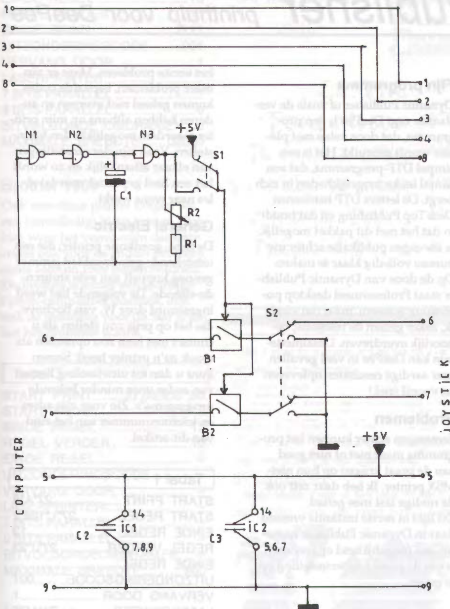
SCHEMA VAN HET AUTOFIRE-MODUL
