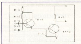
Fig. 3 - Circuito eletrônico de uma porta NAND. TR-1 e TR-2 são tipo 2N2222. Os diodos são do tipo IN914 e os resistores de 2.000 ohms, 1/8 de watt. Bastam entre uma e três centenas destas portas a Máquina Speculatrix MSX 3.0.
