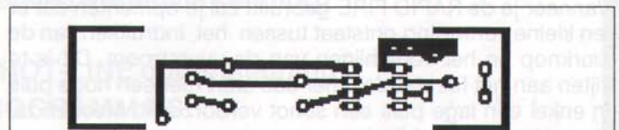
Fig. 3 - De printlayout voor het Rapid fire-circuit (ongeveer ware grootte), met zicht op de koperzijde.
