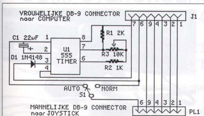
Fig. 2 - Dit schematische diagram laat het hart van het Rapid Fire circuit zien, een CMOS 555 oscillator/timer IC, dat geschakeld is als een astabiele multivibrator, geactiveerd door de gebruiker.
